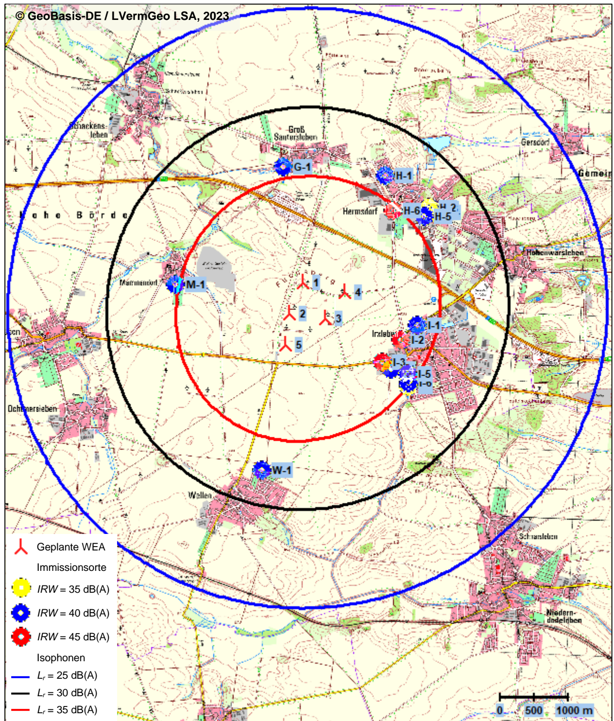
Abbildung 2: Einwirkungsbereich Zusatzbelastung (Nachtbetrieb)
