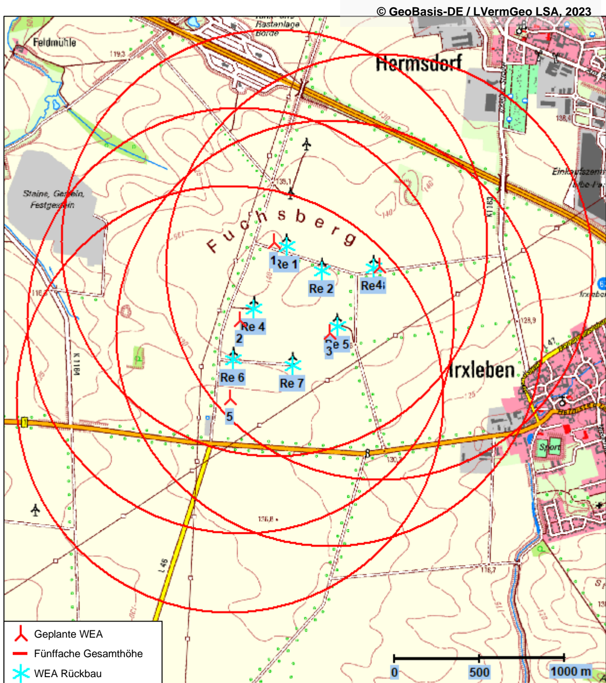
Abbildung 12: Fünffacher Gesamthöhenabstand WEA-Planung
