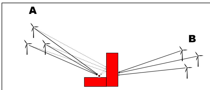
Abbildung 11: Lagekonstellation (Beispiel) – Reflexion von A, Abschirmung von B
